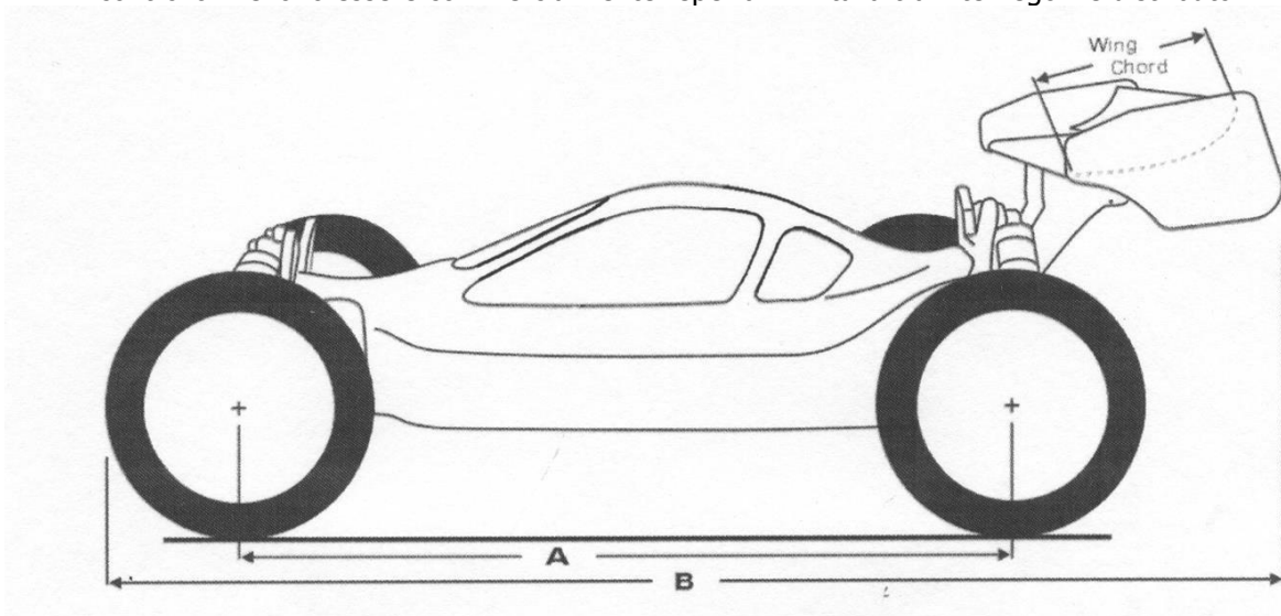
Figura 12: Dimensioni principali 1/8 Brushless
